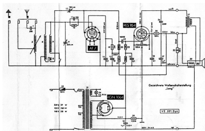
המעגל החשמלי של דגם VE301Dyn
